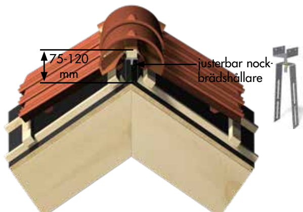
Bild 4. Här används med fördel vår justerbara nockbrädhållare.
