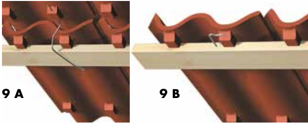
Bild 9. Montering av Benders JP-krok resp takpannekrok.
