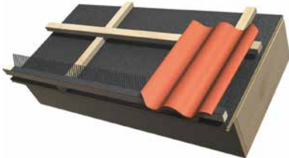
Bild 11. Fågelbandet monteras på takfotsläkten. (Takfotsläkten ska vara ca 10 mm högre än bärläkten, se bild 2).
